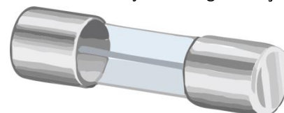
Napięcie: 250V Prąd: 10A Średnica: 5mm Wysokość: 20mm
